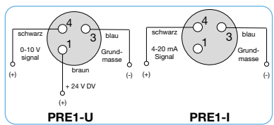
Anschlussplan
